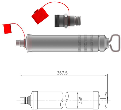
前端补脂枪套件
