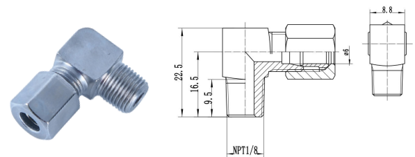
直角卡套接头
