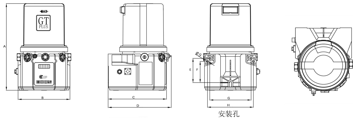
2L&4L 安装尺寸 (单位: mm)
