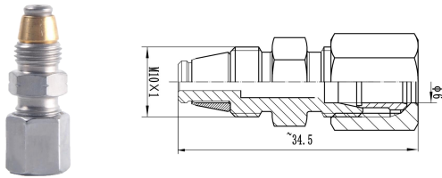
直通卡套接头 带锥度密封/带止回阀
