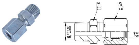
直通卡套接头
