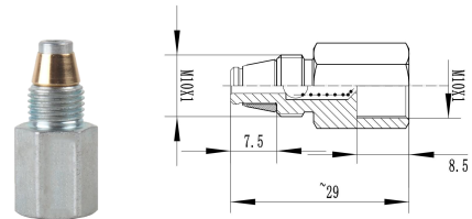
直通接头 带锥度密封/带止回阀
