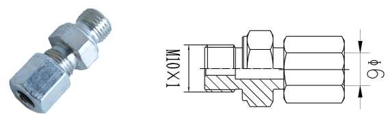
直通卡套接头 带止回阀
