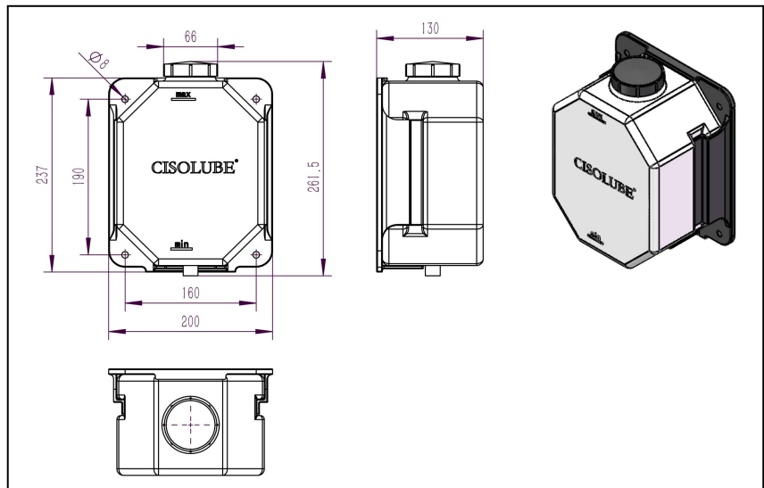
7L 油箱, 带滤芯
