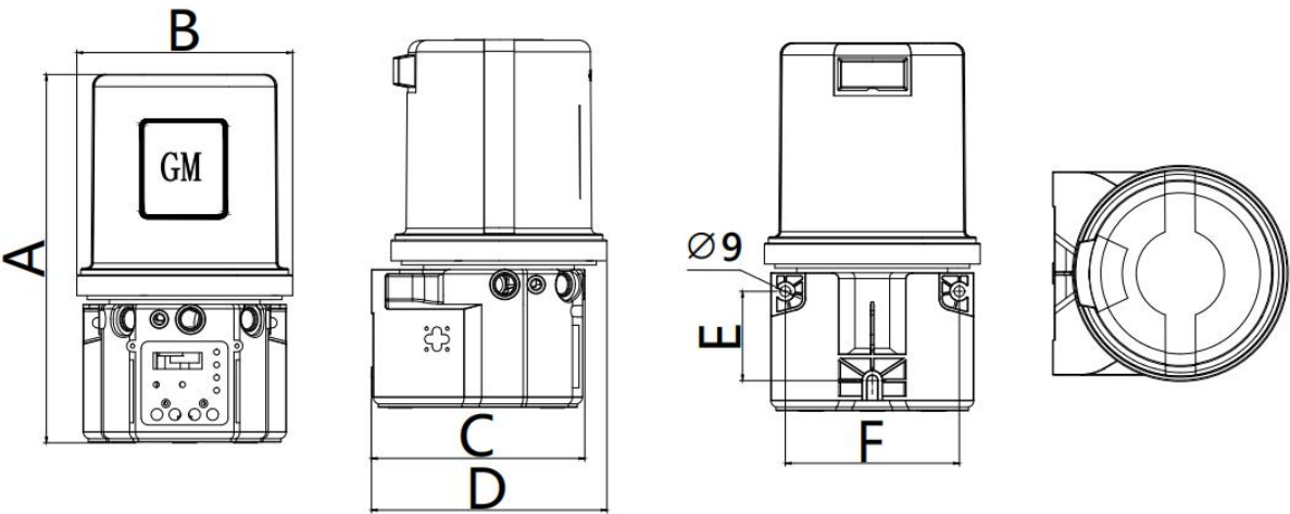
2L&4L 安装尺寸 (单位: mm)
