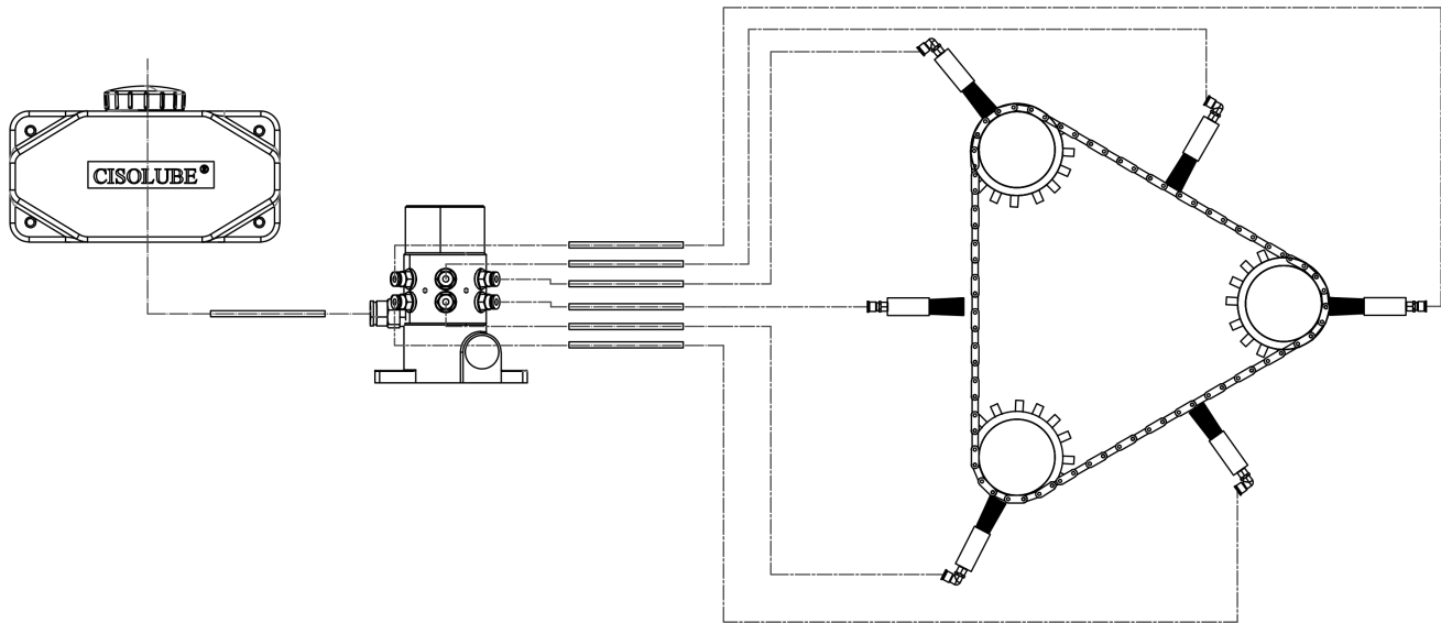
系统示例图
